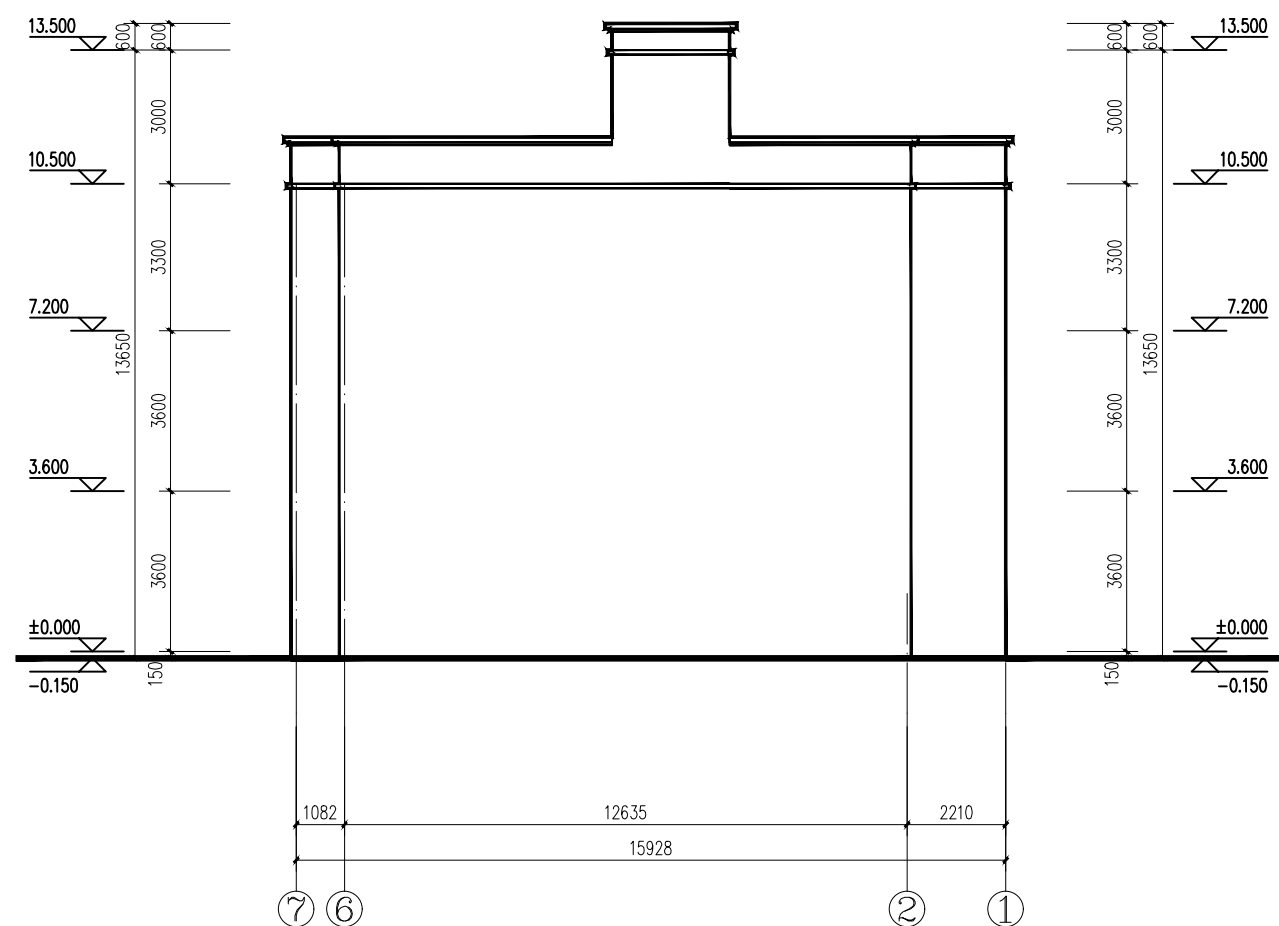
⑦-①轴立面图 1:100
