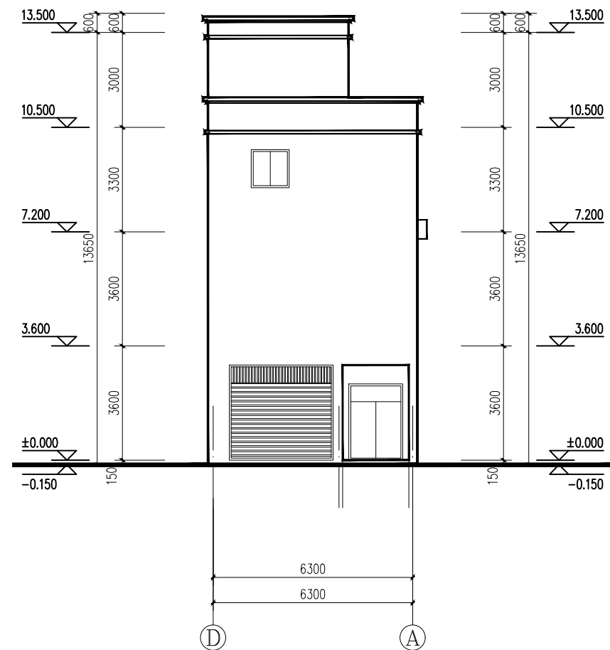
E-A轴立面图 1:100
