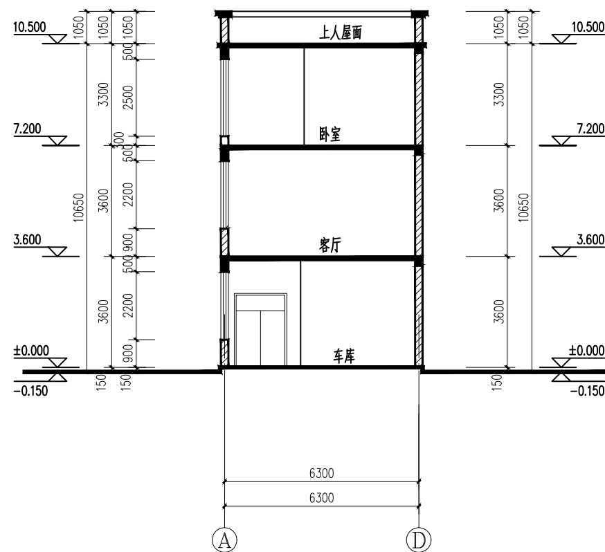
1-1剖面图 1:100
