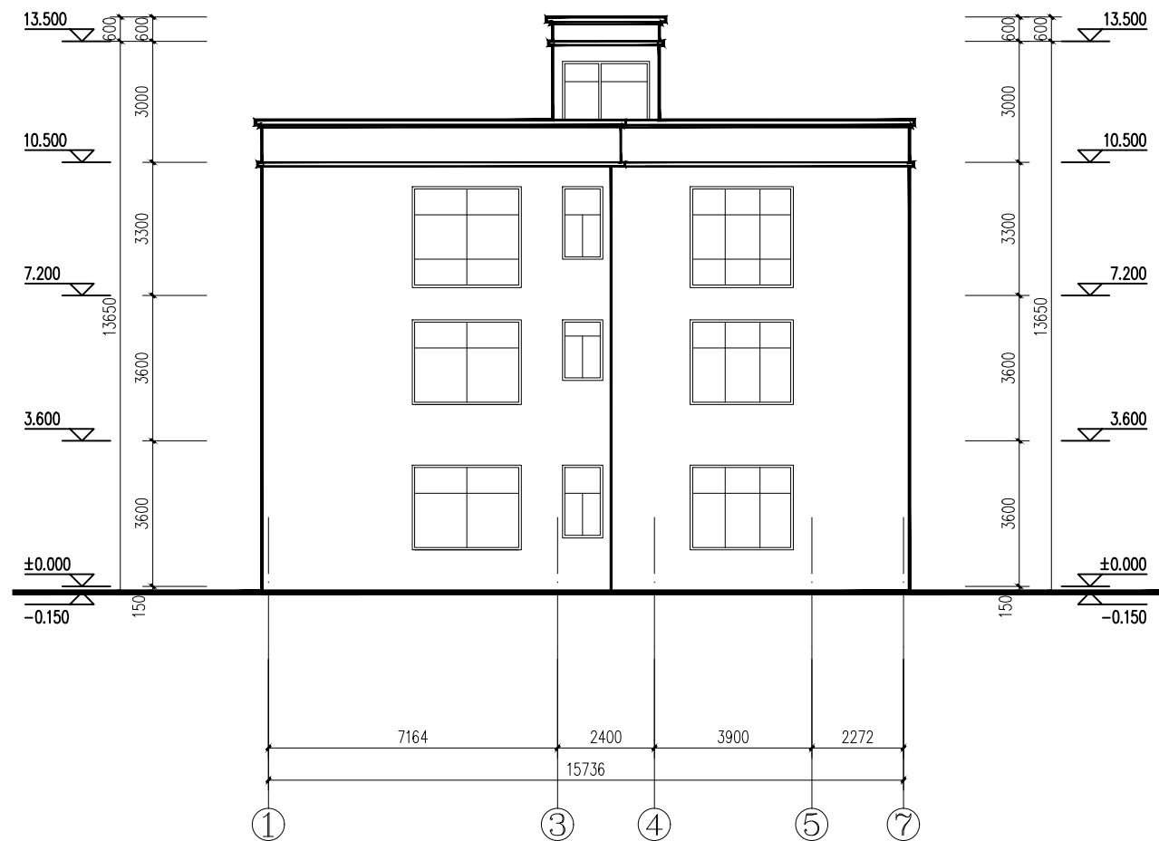
①-⑦轴立面图 1:100
